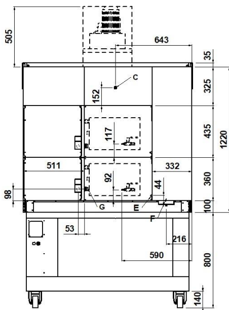
VISTA POSTERIORE
