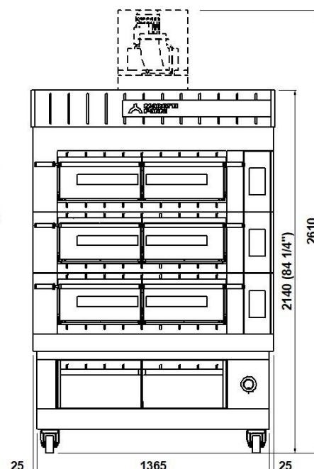
VISTA FRONTALE
