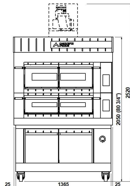
VISTA FRONTALE
